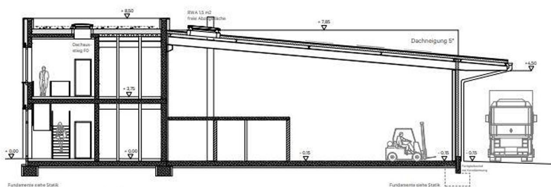
Schnitt A-A
