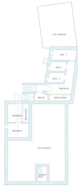
Kellergeschoss 1 100
