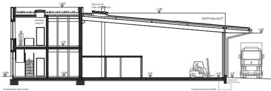
Schnitt A-A
