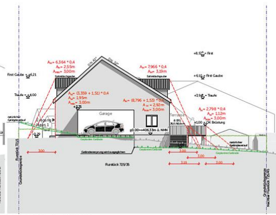
Ansicht West - M1:100
