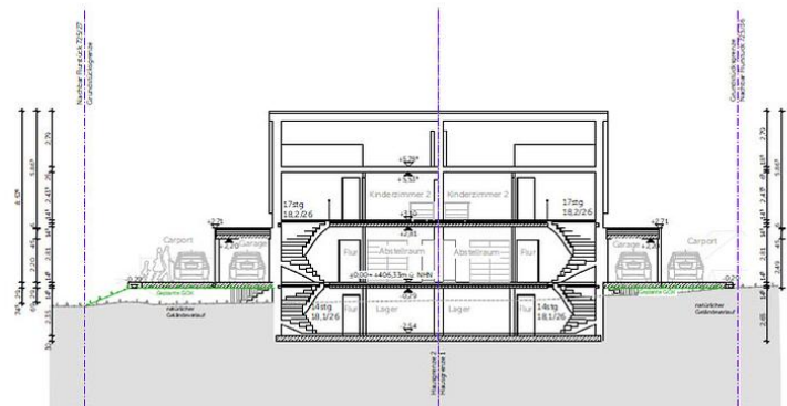
Schnitt A-A - M1:100
