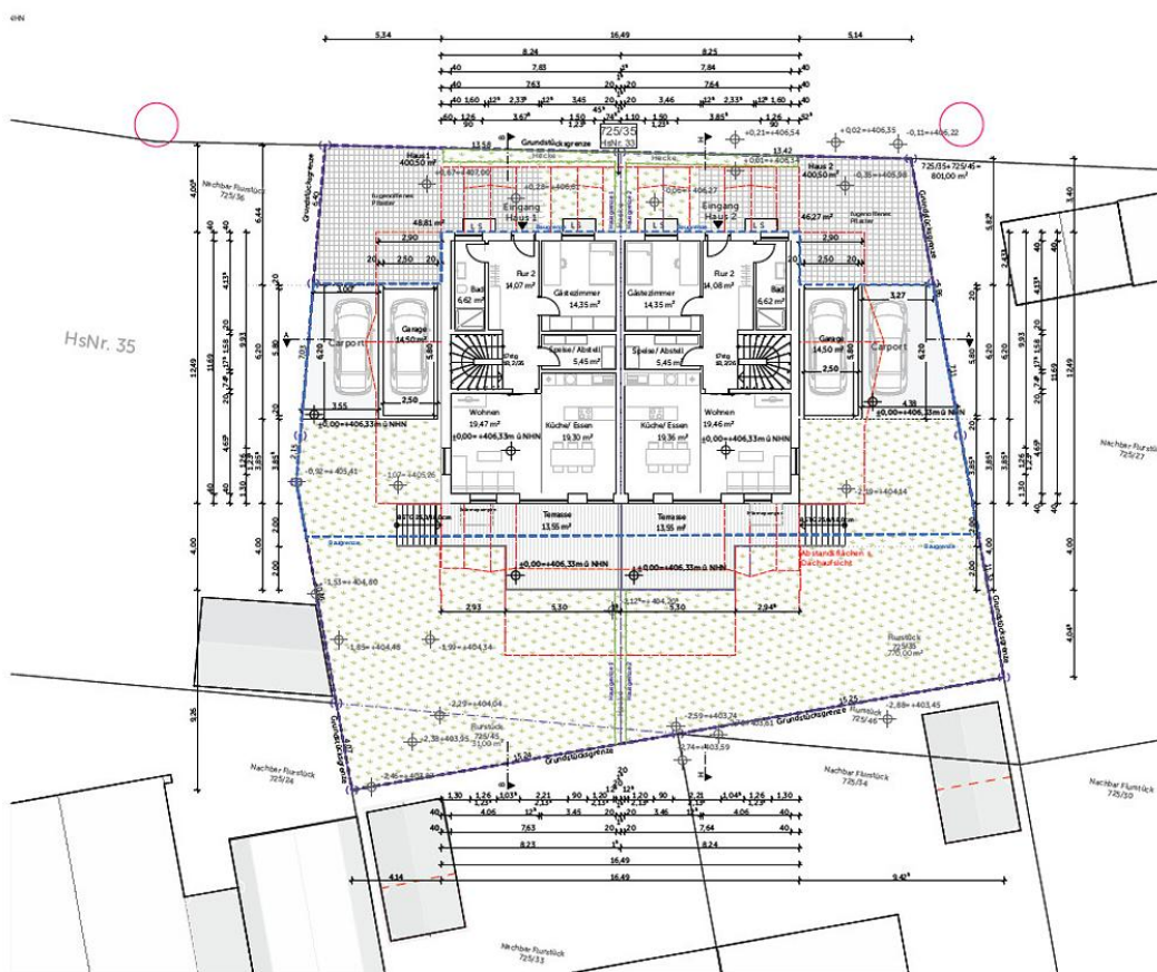
Erdgeschoss - M1:100
