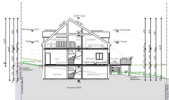
Schnitt H-H - M1:100
