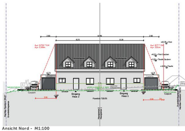
Ansicht Nord - M1:100
