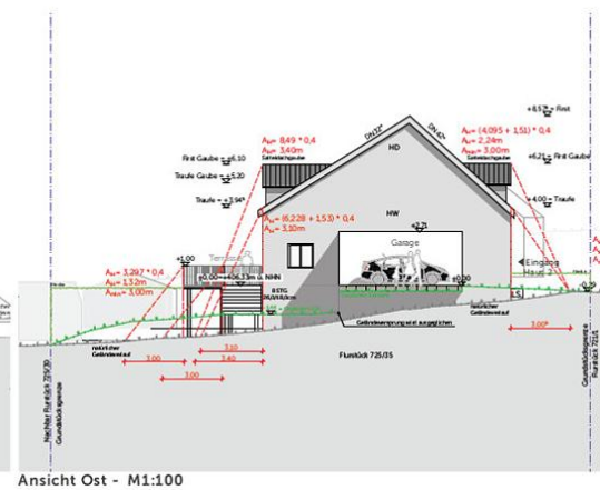
Ansicht Ost - M1:100
