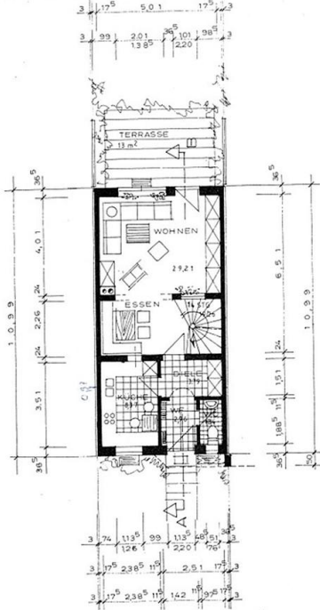
ERDGESCHOSS M. 1 : 1 0 0
