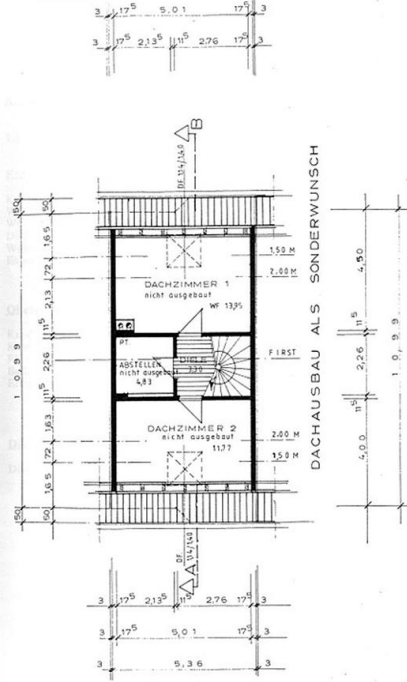
DACHGESCHOSS M. 1 : 1 0 0
