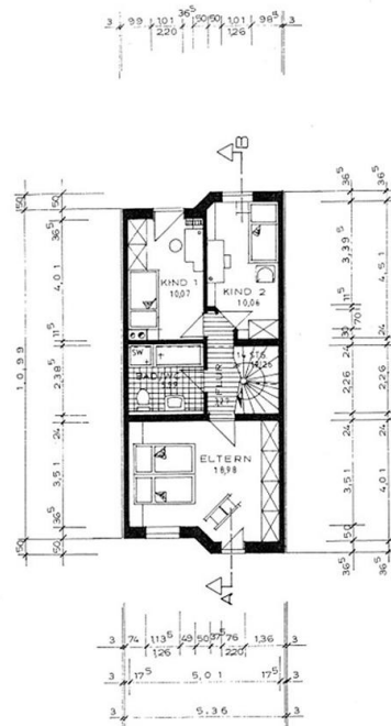
OBERGESCHOSS M. 1 : 1 0 0
