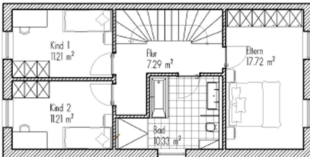
GRUNDRISS OBERGESCHOSS
